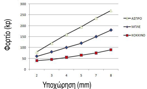
Διάγραμμα Φόρτισης
